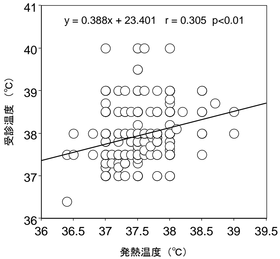
図 6 . 発熱温度と受診温度との関係
